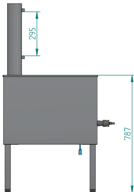
VISTA LATERAL
