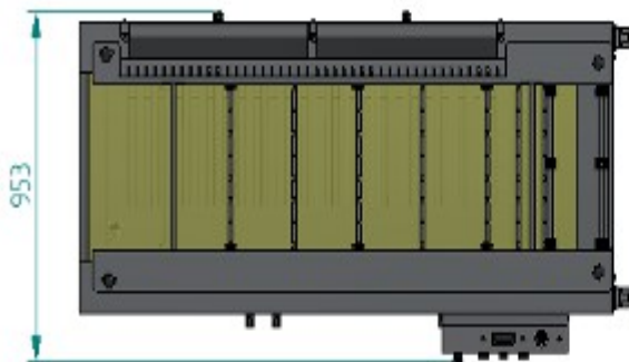
VISTA PLANTA
