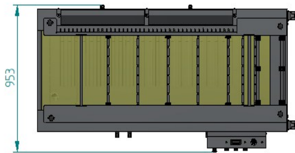
VISTA PLANTA
